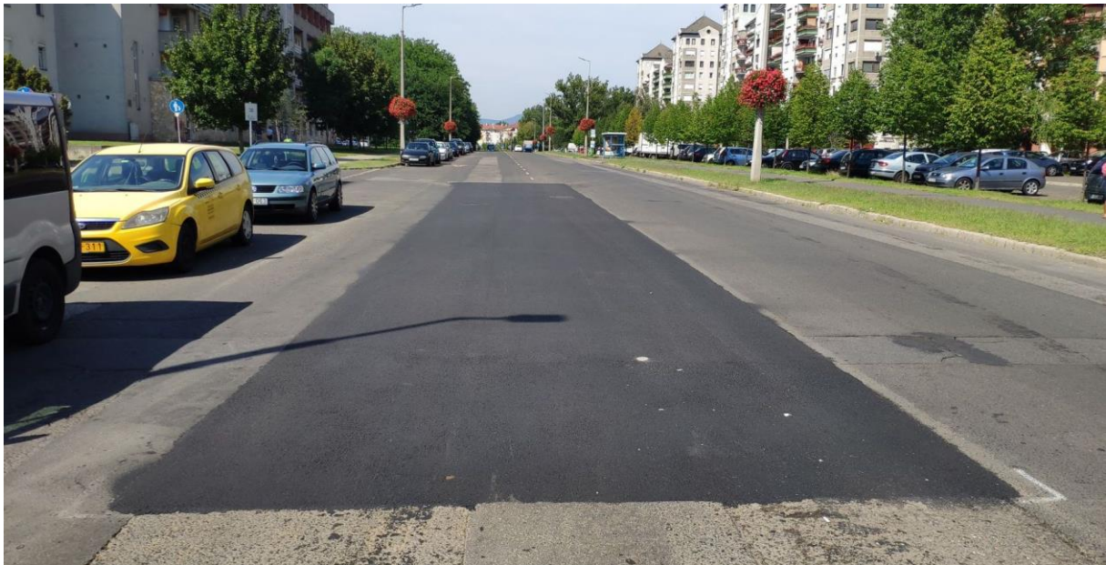
IV. kerület Megyeri út 203. – egyrétegű aszfaltjavítás 129 négyzetméteren
